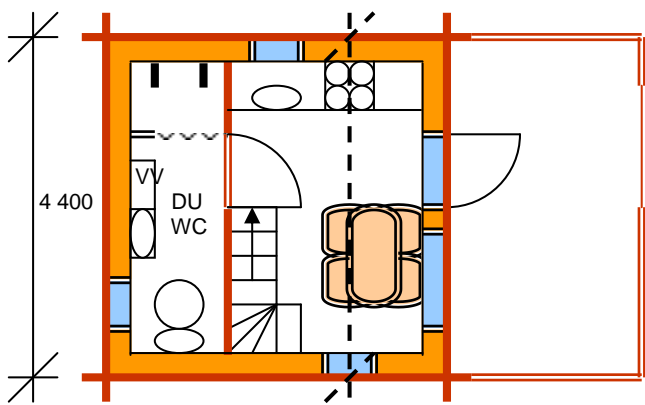
SEKTION AA
