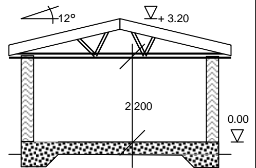
SEKTION AA
