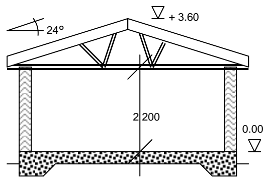
SEKTION AA
