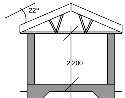
SEKTION AA
