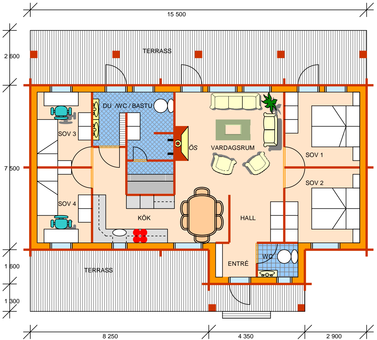
PLANLÖSNING
